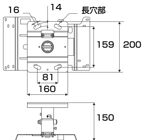
天井接地面寸法図（単位：mm）
