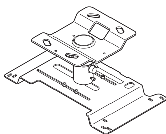
Staffa di montaggio a soffitto ELPMB22
